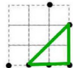
Triangle rectangle isocèle
