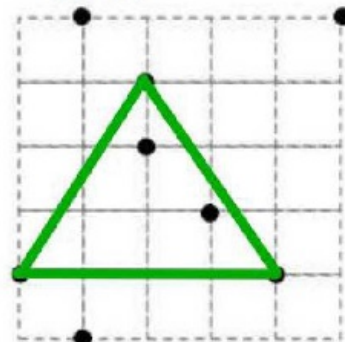
Triangle rectangle isocèle
