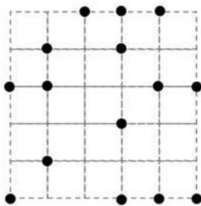
Losange
