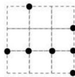
Parallélogramme
