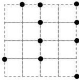
Carré
