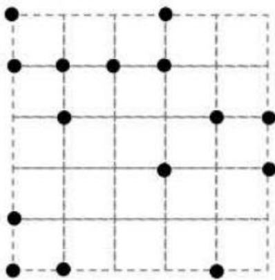
Carré
