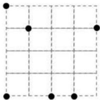
Triangle isocèle
