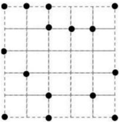
Carré
