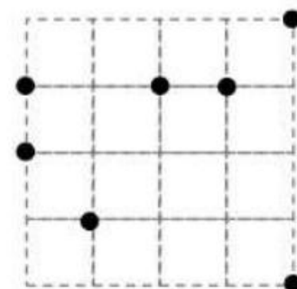
Trapèze
