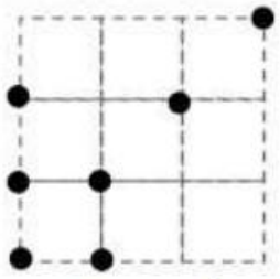
Carré
