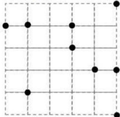
Parallélogramme
