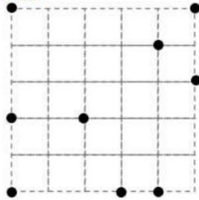
Parallélogramme
