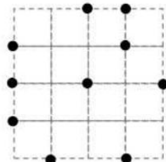
Losange
