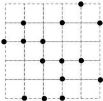
Losange
