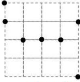
Triangle isocèle
