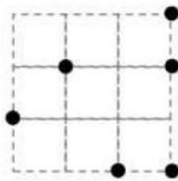
Trapèze
