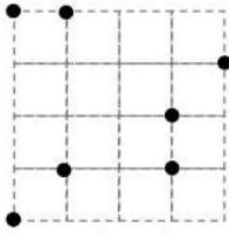
Triangle isocèle
