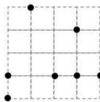
Trapèze
