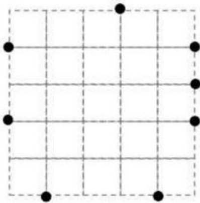
Triangle isocèle
