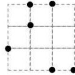
Parallélogramme
