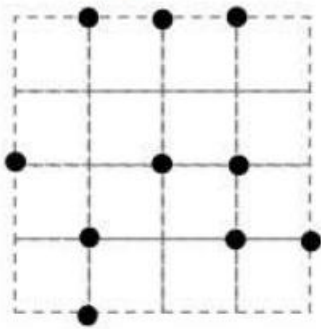
Losange
